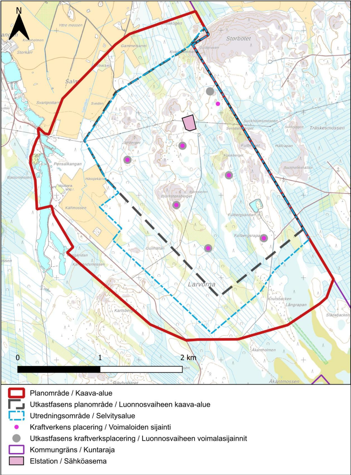
Kuva 1. Kaavaluonnoksen ja kaavaratkaisun tuulivoimalasijainnit (7 voimalaa) 17.4.2026
